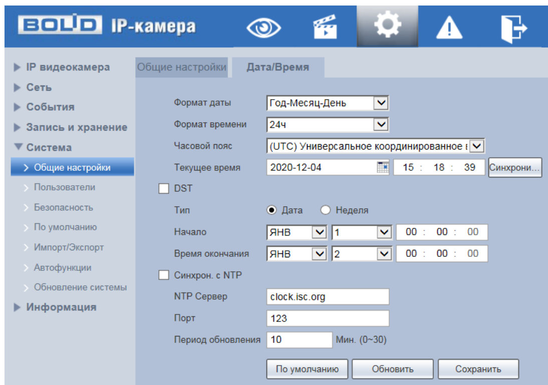
Рисунок 7.109 – Вкладка «Дата/Время»
