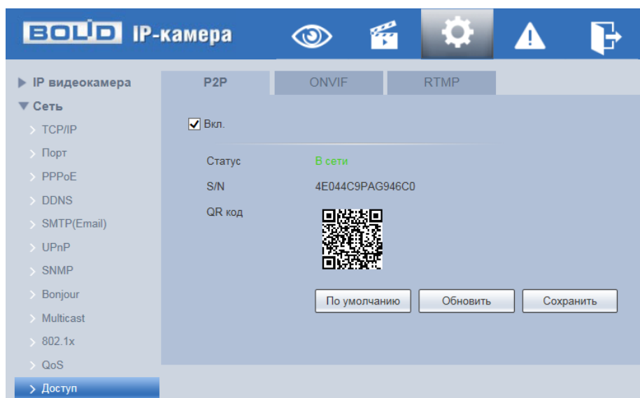
Рисунок 7.67 – Вкладка «P2P»
