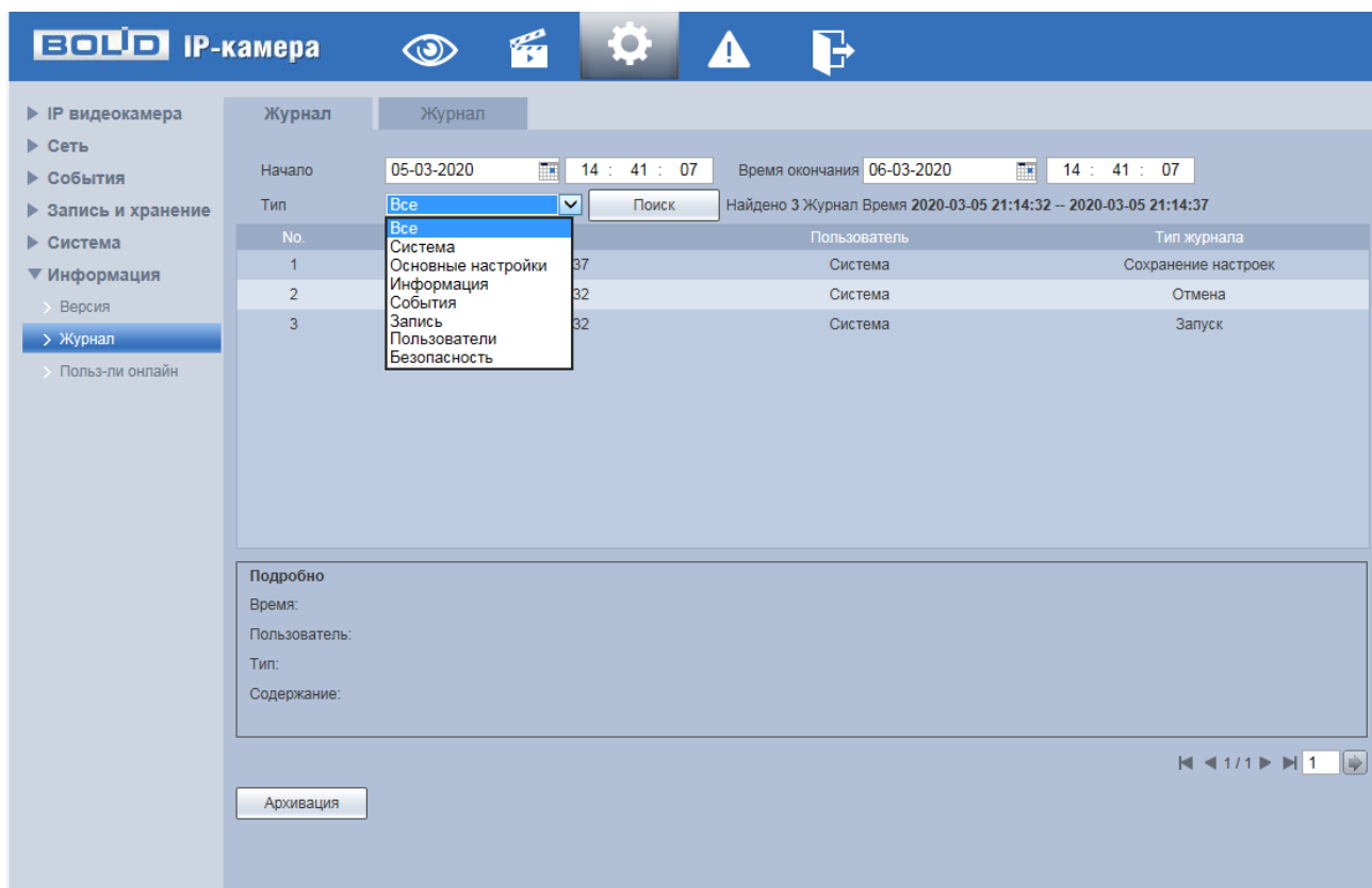
Рисунок 7.126 – Вкладка «Журнал»
