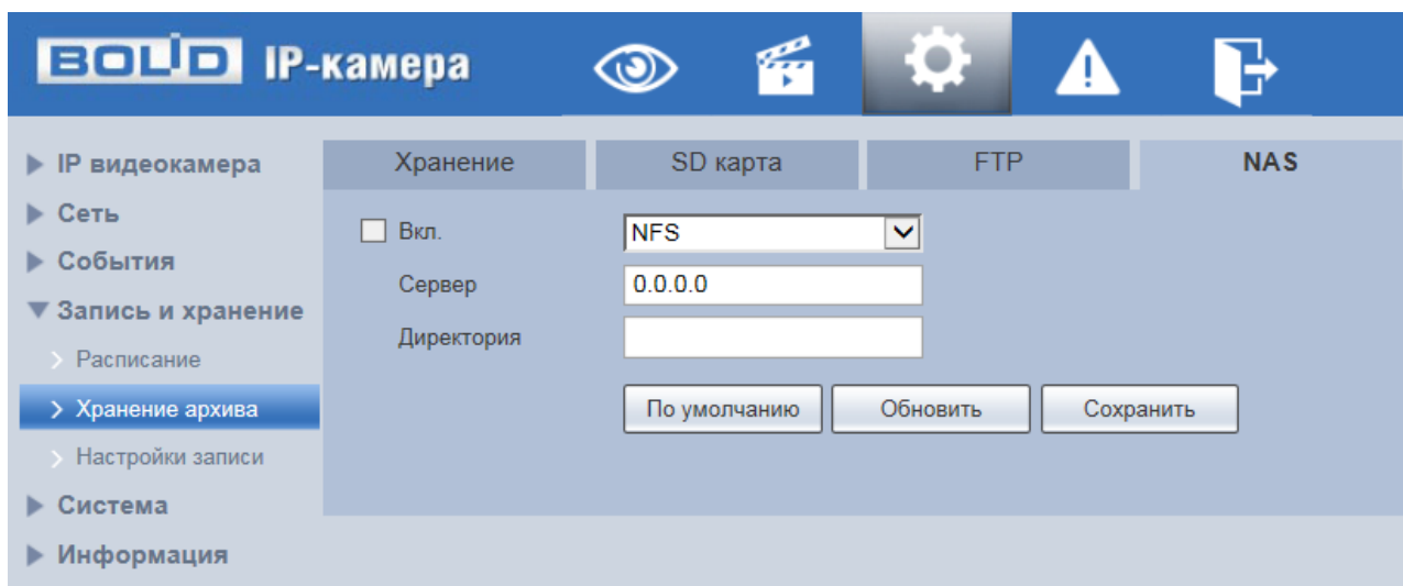
Рисунок 7.103 – Вкладка «NAS»
