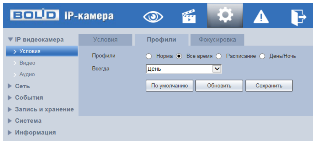
Рисунок 7.36 – Вкладка «Профили»
