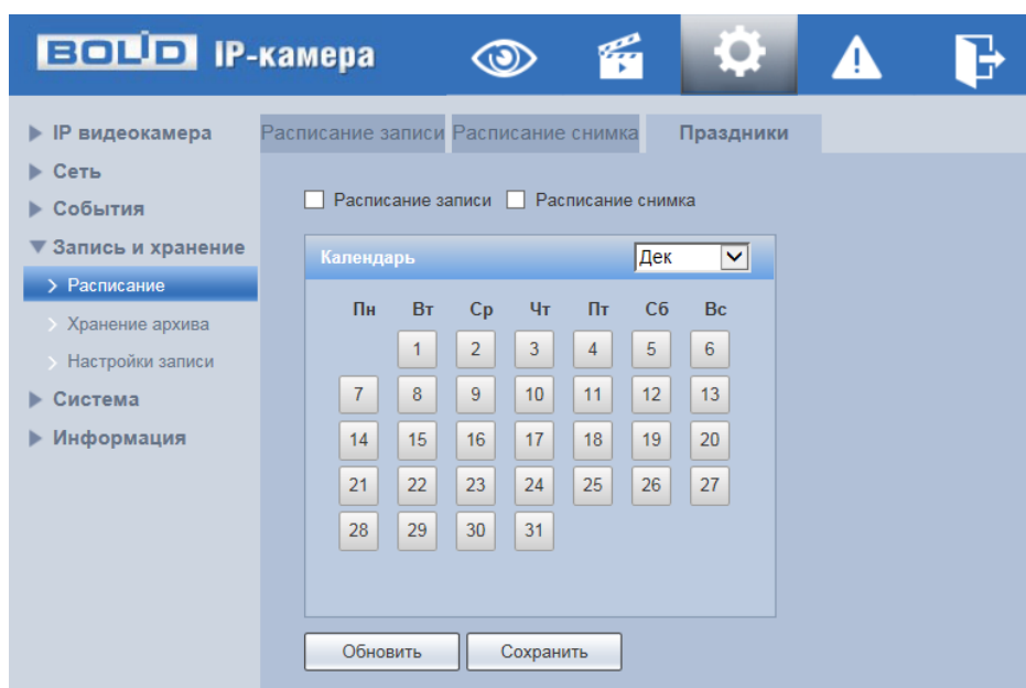
Рисунок 7.98 – Вкладка «Праздники»
