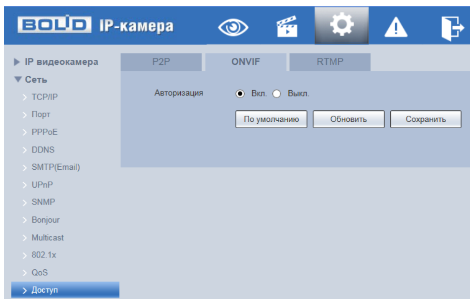
Рисунок 7.68 – Вкладка «ONVIF»
