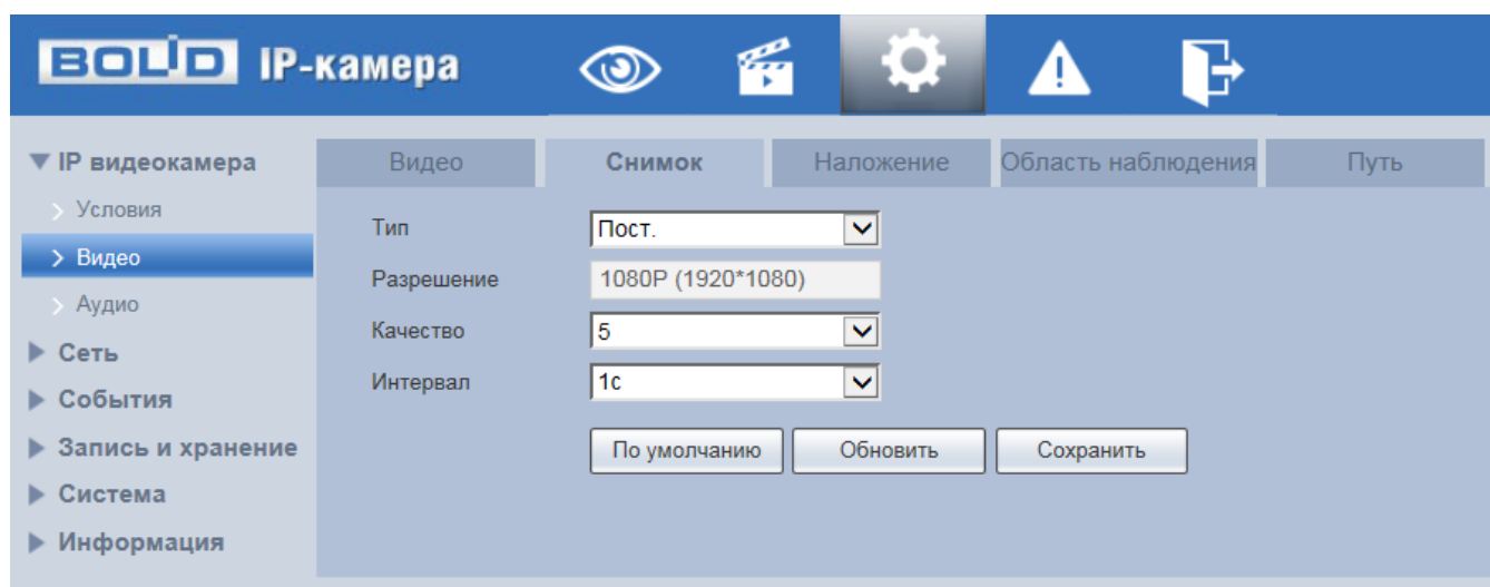
Рисунок 7.40 – Вкладка «Снимок»
