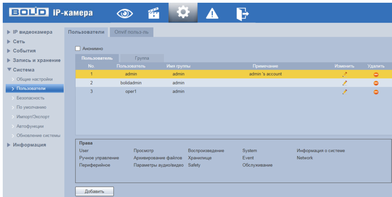
Рисунок 7.111 – Вкладка «Пользователи»
