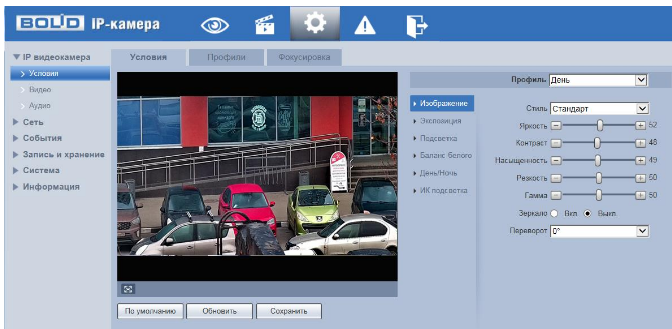
Рисунок 7.27 – Вкладка «Условия»
