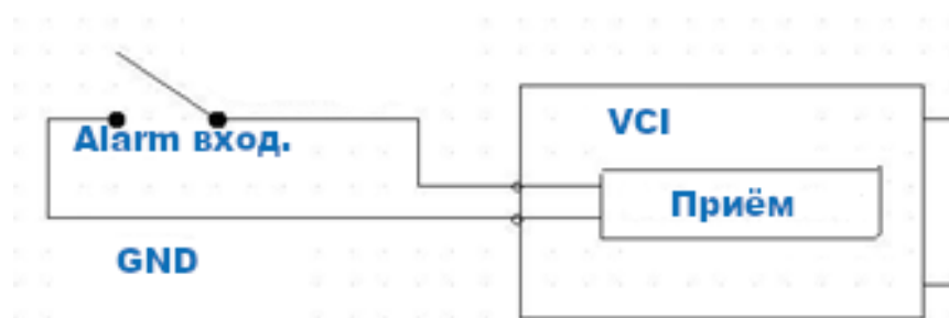
Рисунок 6.13 – Схема подключения тревожного входа
