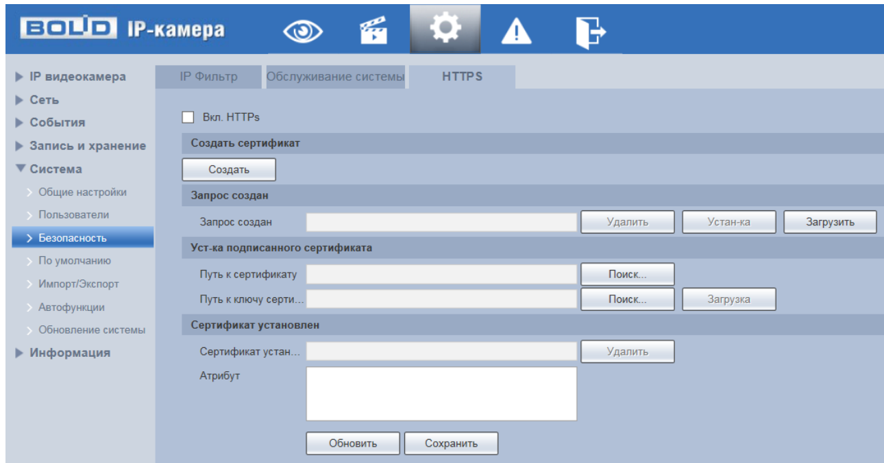
Рисунок 7.117 – Вкладка «HTTPS»
