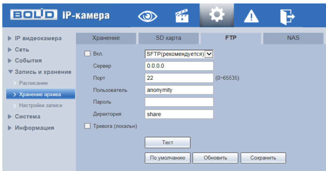
Рисунок 7.102 – Вкладка «FTP»
