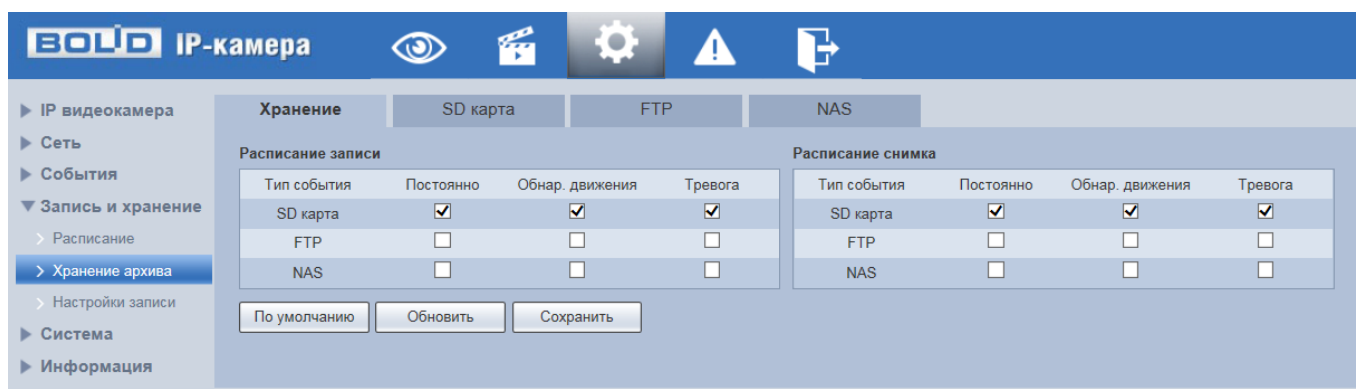
Рисунок 7.100 – Вкладка «Хранение»
