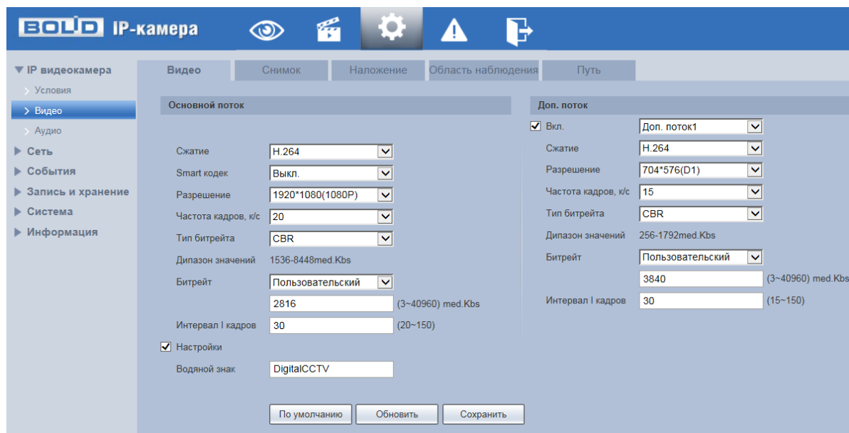
Рисунок 7.39 – Вкладка «Видео»
