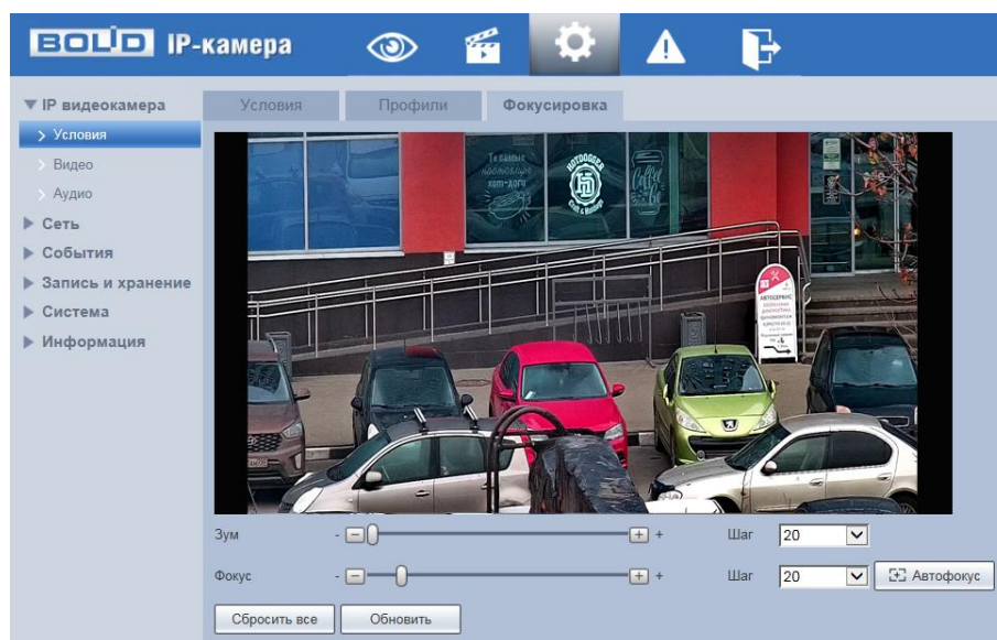
Рисунок 7.37 – Вкладка «Фокусировка»
