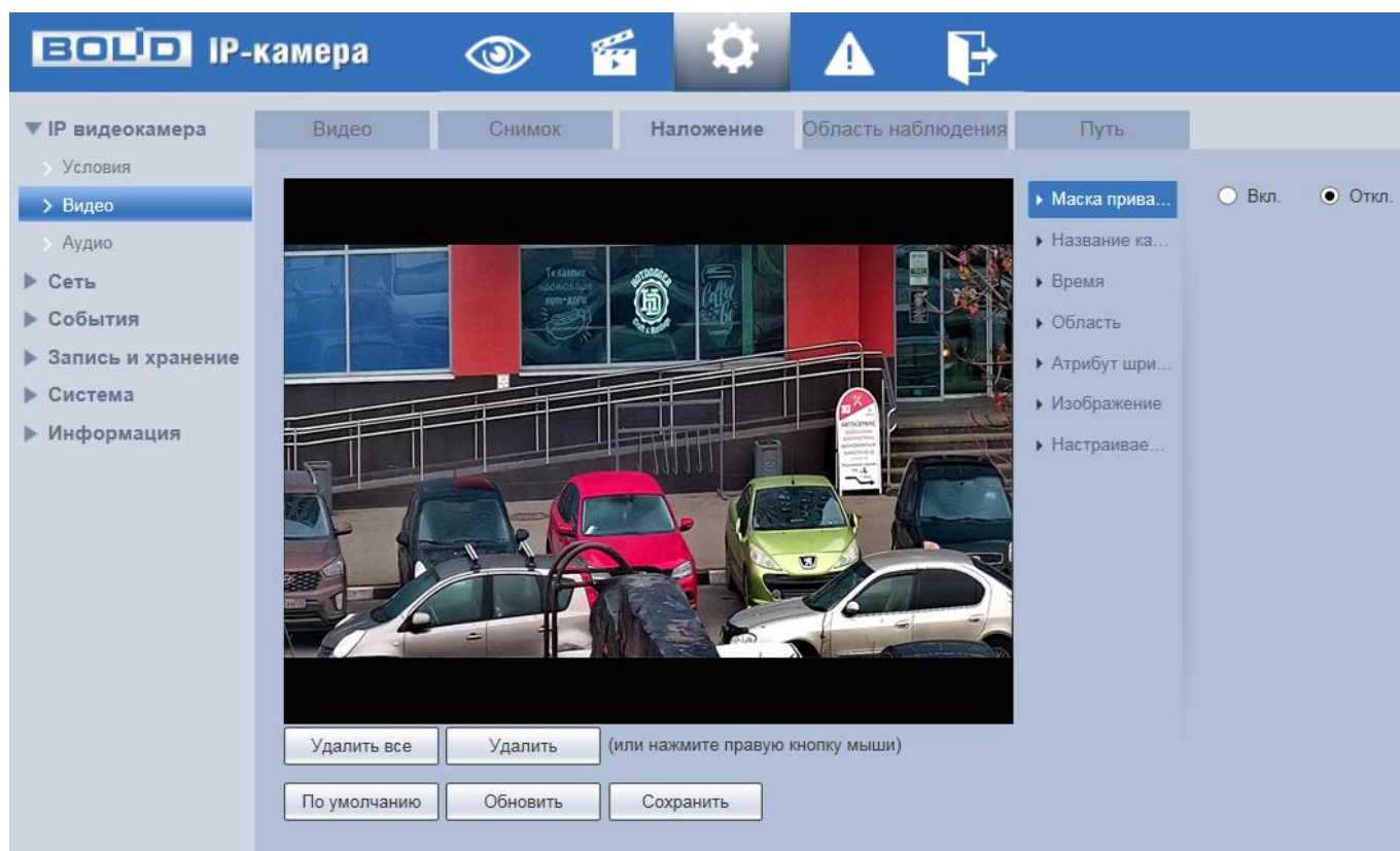
Рисунок 7.41 – Вкладка «Наложение»
