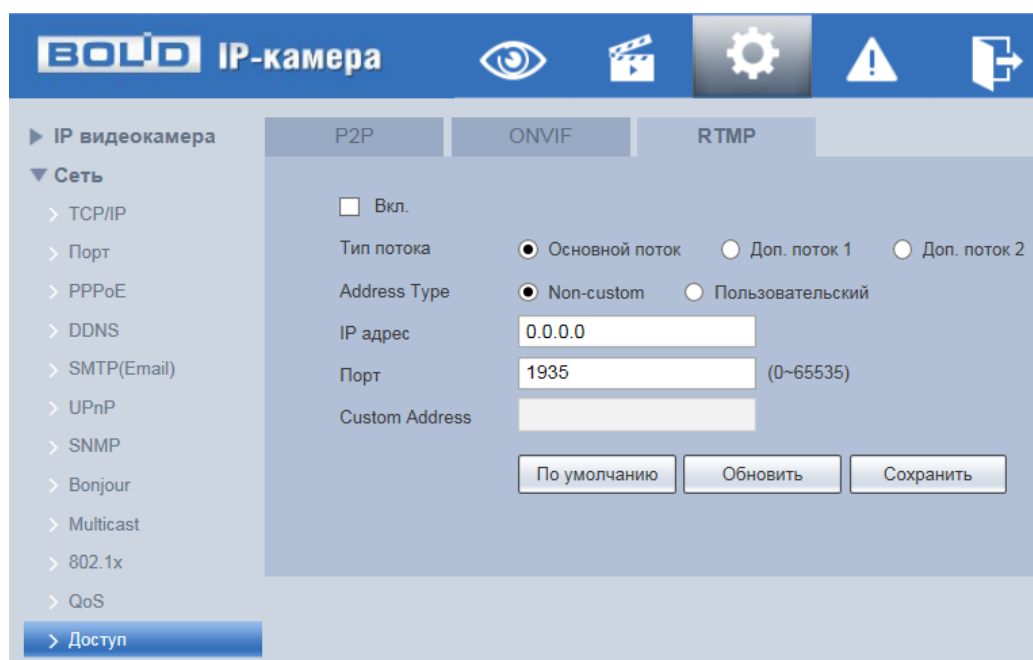
Рисунок 7.69 – Вкладка «RTMP»
