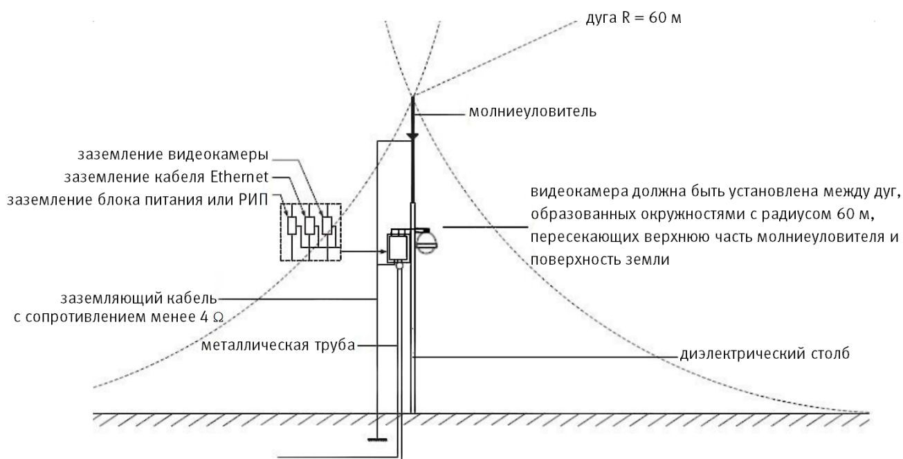
Рисунок 6.14 – Установка молниеотвода
