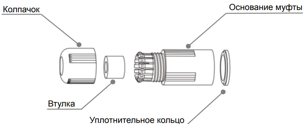
Рисунок 6.6 – Элементы герметичной кабельной муфты
